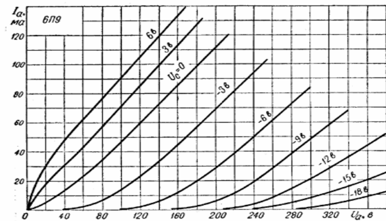
Рис. 403. Усредненные характеристики зависимости тока анода от напряжения на аноде в триодном включении.
