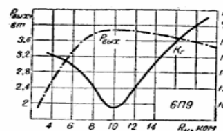
Рис. 404. Усредненные характеристики зависимости выходной мощности и коэффициента нелинейных искажений от сопротивления нагрузки при напряжении на аноде 300 в, напряжении на второй сетке 150 в, напряжении смещения на первой сетке — 3 в и переменном напряжении на первой сетке 2,1 в эф.
