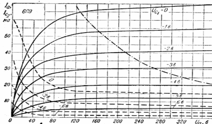
Рис. 403. Усредненные характеристики зависимости тока анода и тока второй сетки от напряжения на аноде при напряжении на второй сетке 150 в: — ток в цепи анода; — ток в цепи второй сетки; — наибольшая мощность, рассеиваемая на аноде.
