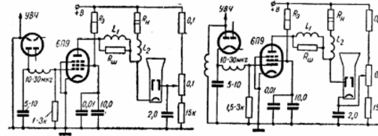
Рис. 399. Схема применения лампы 6П9 для работы в режимах I—III.
