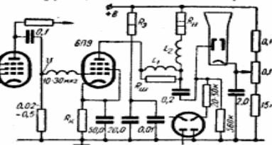
Рис. 402. Схема применения лампы 6П9 для работы в режиме VIII.
