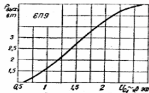
Рис. 405. Динамическая характеристика зависимости выходной мощности от переменного напряжения сигнала на первой сетке.
