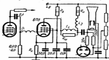
Рис. 401. Схема применения лампы 6П9 для работы в режимах VI и VII.
